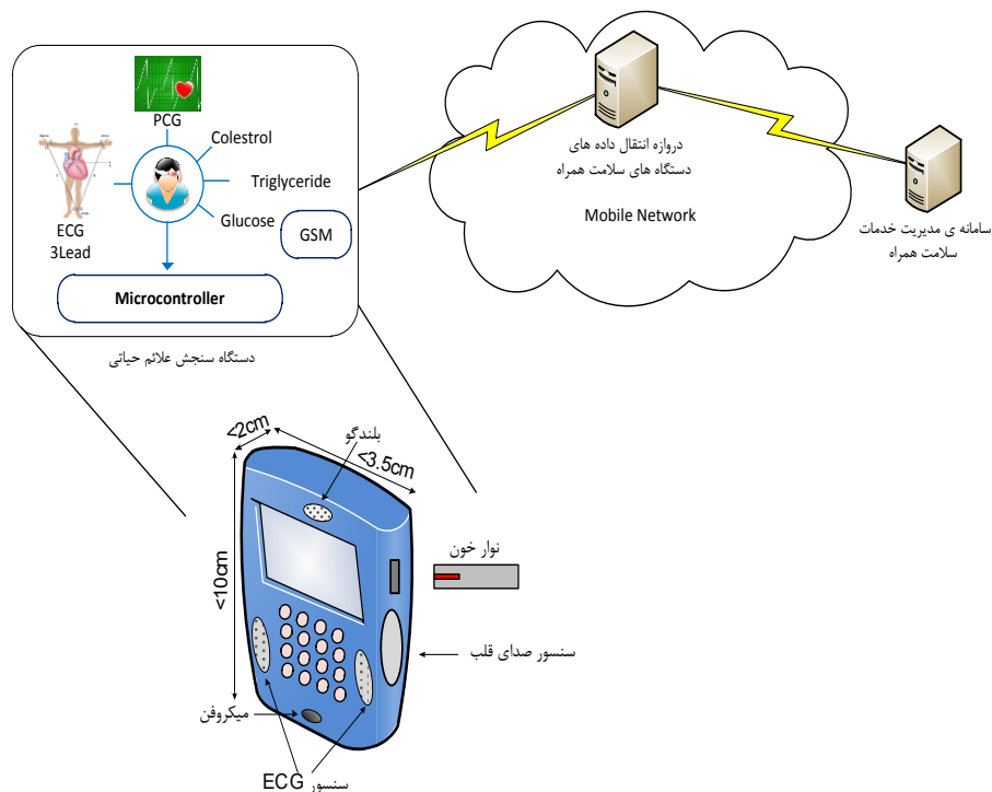
شکل ۲- نمای کلی ارتباط اجزای پروژه‌ی "نظارت و سنجش از راه دور علائم حیاتی"
