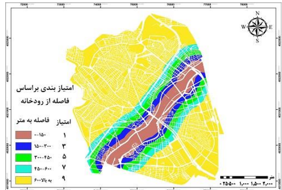
شکل ۸. نقشه امتیازدهی شده شاخص رودخانه
